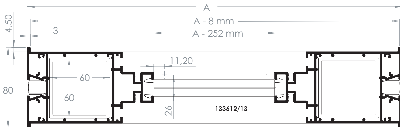
139738 Boormat T-verbinder [133612/13] Bohrschablone T-Verbinder Drilling template T-connector
