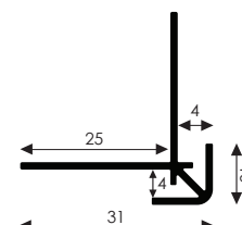
134226 Buitenhoekprofiel 4/4100 anod (+T) External corner 4/4100 anod (+T) Außeneckprofil 4/4100 elox (+T)
